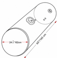
KENWORTH T680 2014 -2022 Tanque Diesel 135 GL 65x24 1/2
